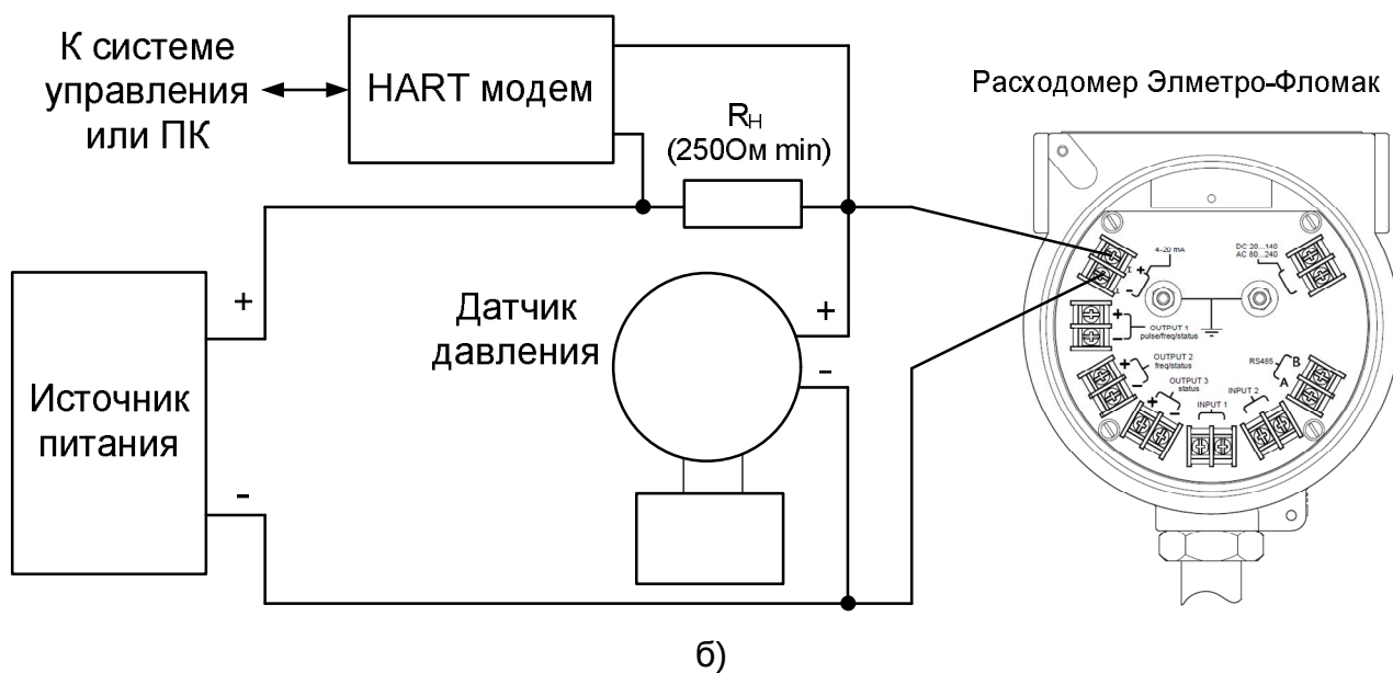
Рисунок В.4 – Подключение датчика давления для компенсации влияния избыточного давления среды на измерение массового расхода и плотности: а) датчик давления работает в монополярном (Burst) режиме; б) датчик давления отвечает на запросы Мастер-устройства (АСУ, коммуникатора или ПК с HART-модемом)
