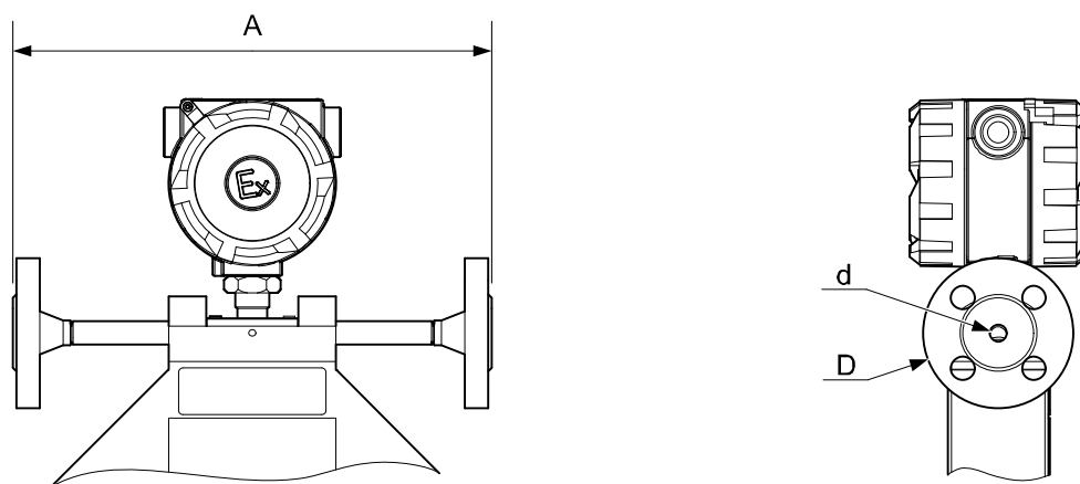
Рисунок Б.3 – Габаритные размеры датчиков S010, S015 с фланцевым присоединением.
