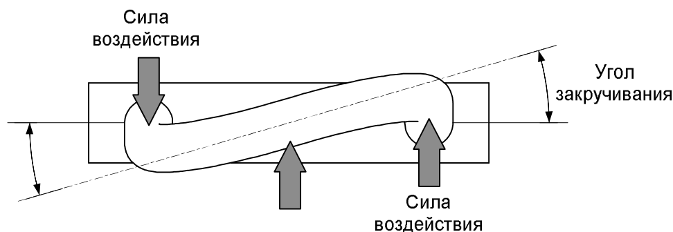
Рисунок 1.9 – Труба датчика и пара сил, приводящая ее к закручиванию
