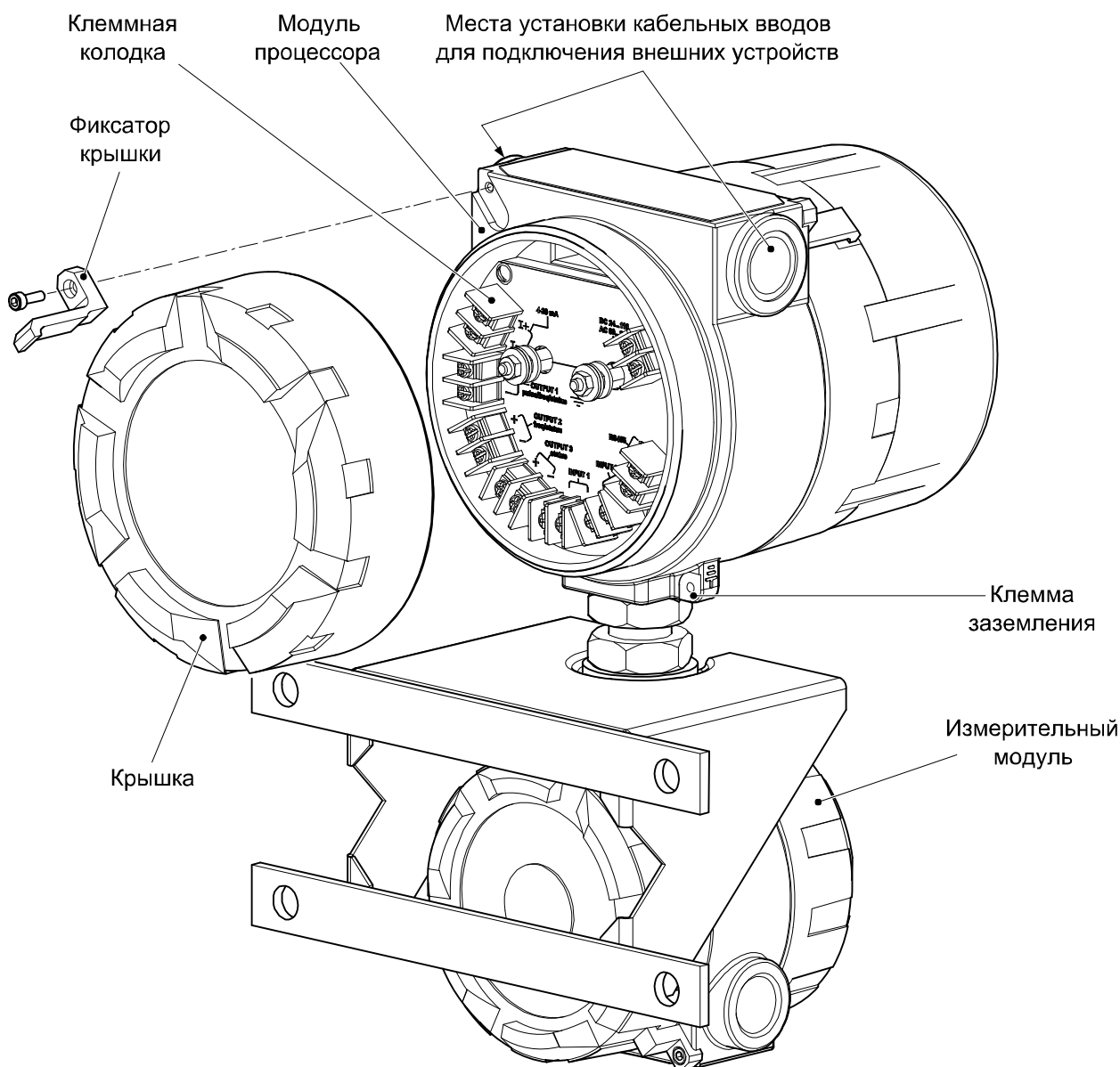
Рисунок 2.11 – Корпус модуля процессора.
