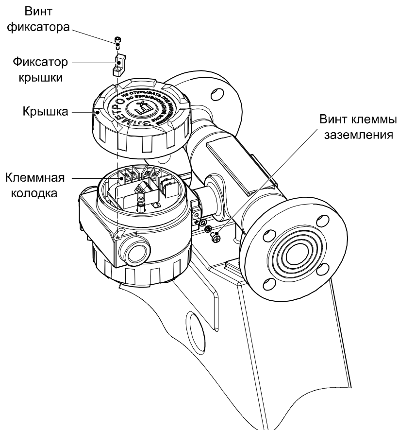
Рисунок 2.5 – Корпус измерительного модуля (исполнения по компоновке I, R) или корпус клеммной коробки 1 (исполнения по компоновке S, RS), размещенный на датчике.
