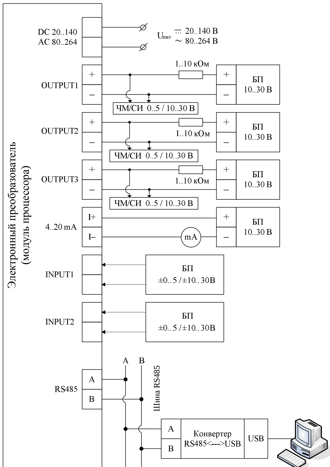
Рисунок В.2 – Схема подключения расходомера к внешним устройствам БП – блок питания, ЧМ – частотомер, СИ – счётчик импульсов, mA – амперметр.
