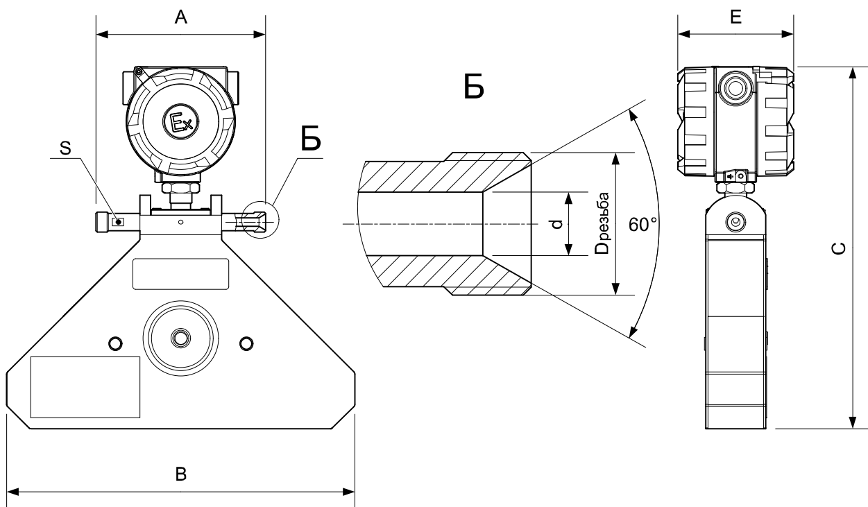
Рисунок Б.2 – Габаритные размеры датчиков S002, S003, S005, S010, S015 со штуцерным присоединением
