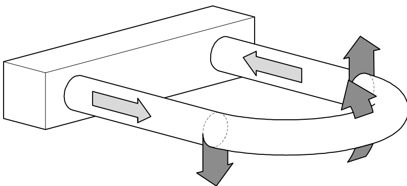
Рисунок 1.8 – Силы, действующие на трубу при движении вверх
