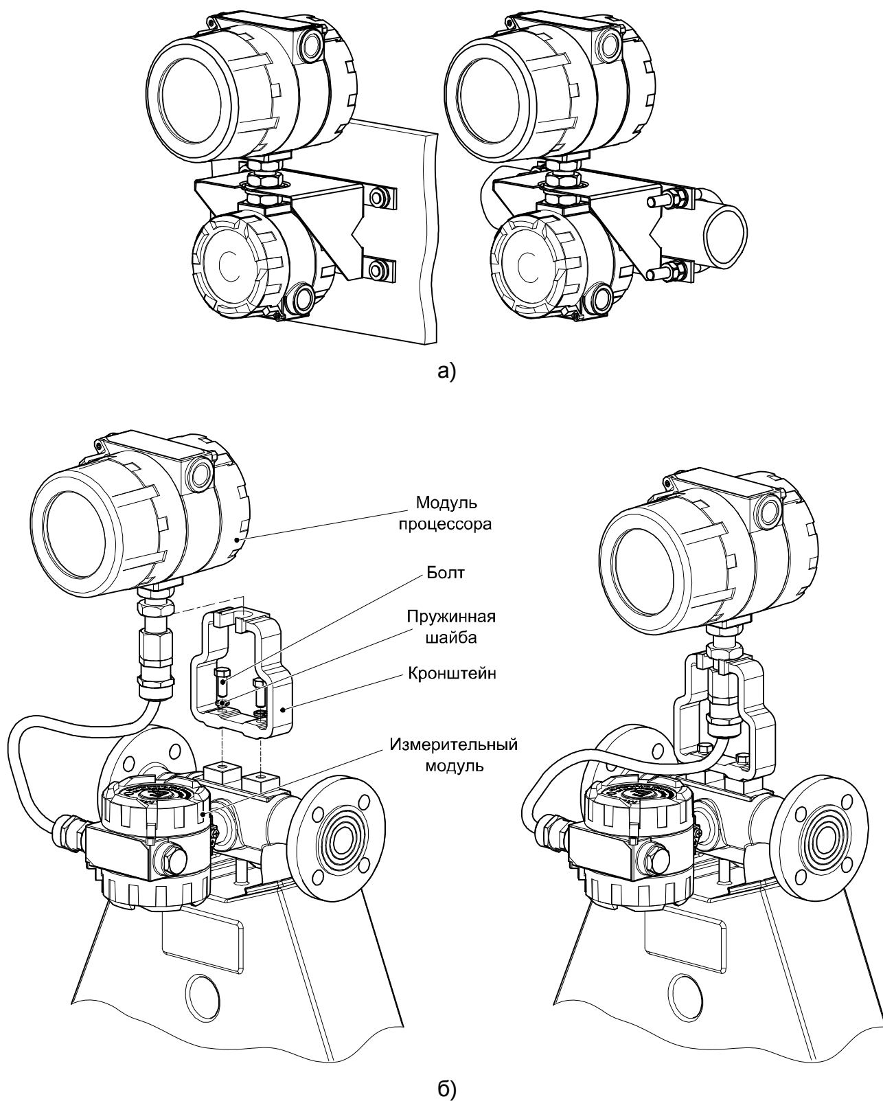
Рисунок 2.10 – Варианты размещения ЭП расходомера.
