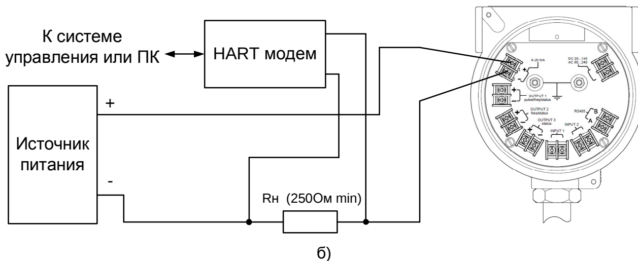
Рисунок В.3 – Схема подключения расходомера к ПК через HART модем. Модем, в зависимости от удобства, подключается к клеммам расходомера (а) или к нагрузочному резистору (б).
