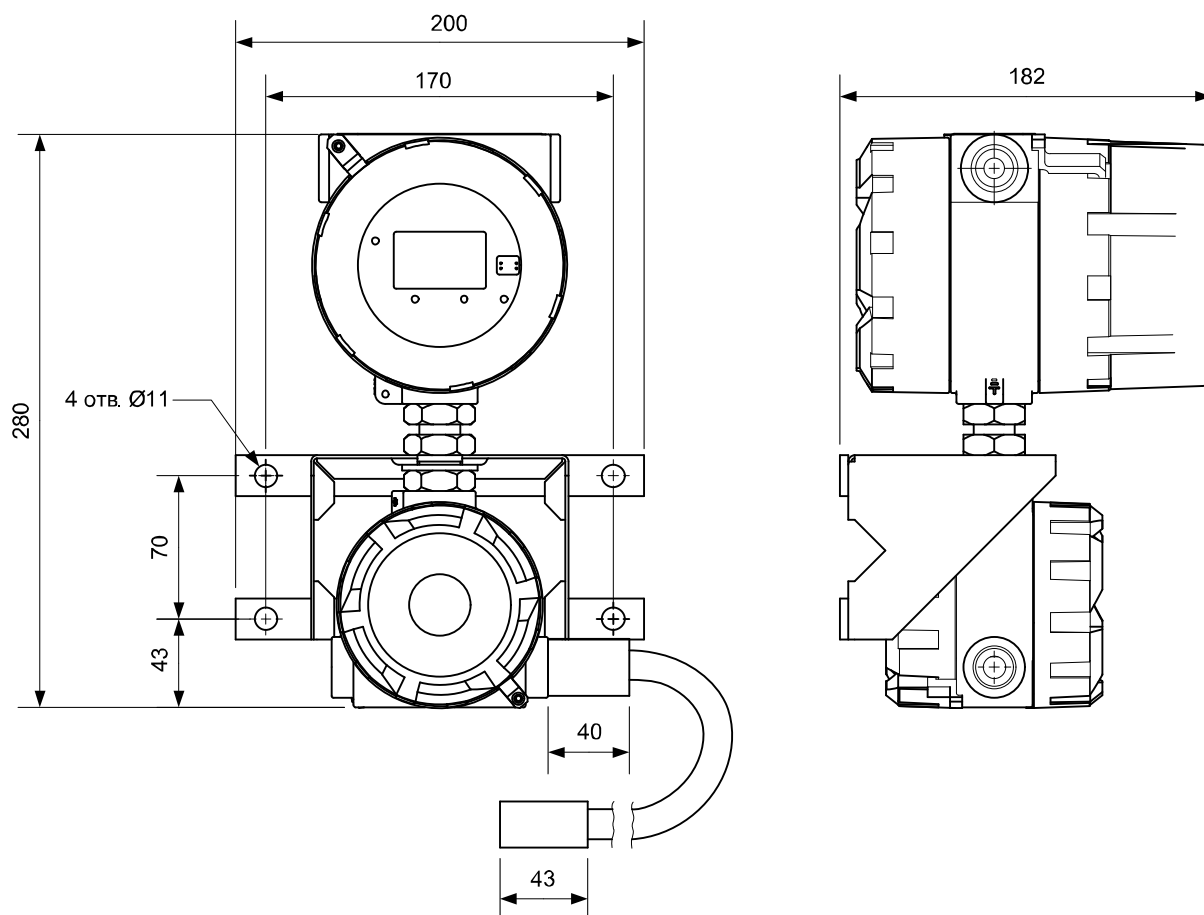
Рисунок Б.4 – Электронный преобразователь (исполнение по компоновке S), модуль процессора (исполнения по компоновке R, RS) на кронштейне.
