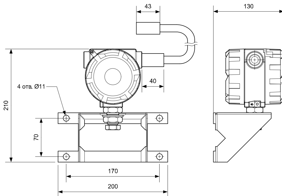
Рисунок Б.5 – Измерительный модуль на кронштейне, исполнение по компоновке RS.
