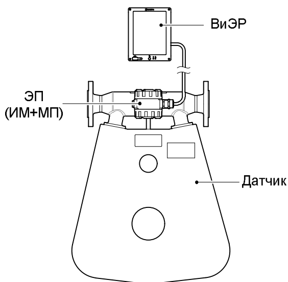
Рисунок 1.6 Компактное исполнение с видеографическим регистратором (V)
