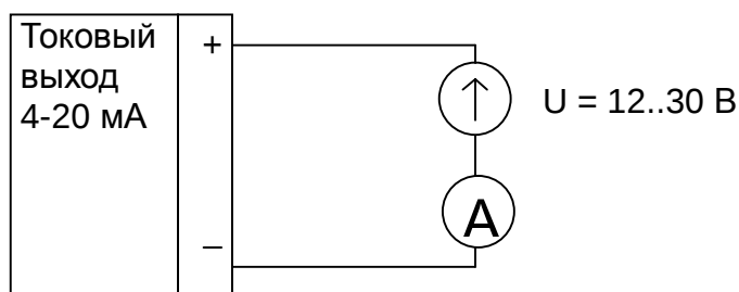
Рис.2.23 Подключение измерителя тока к токовому выходу
