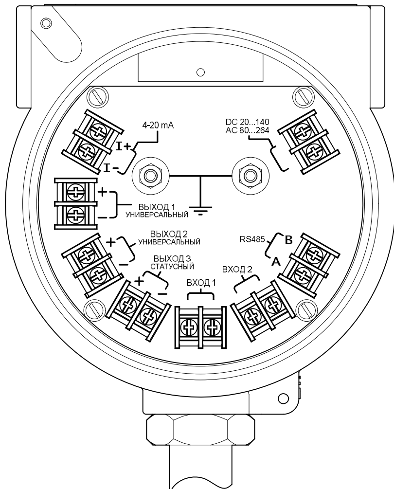
Рисунок В.1 – Размещение присоединительных клемм в модуле процессора.
